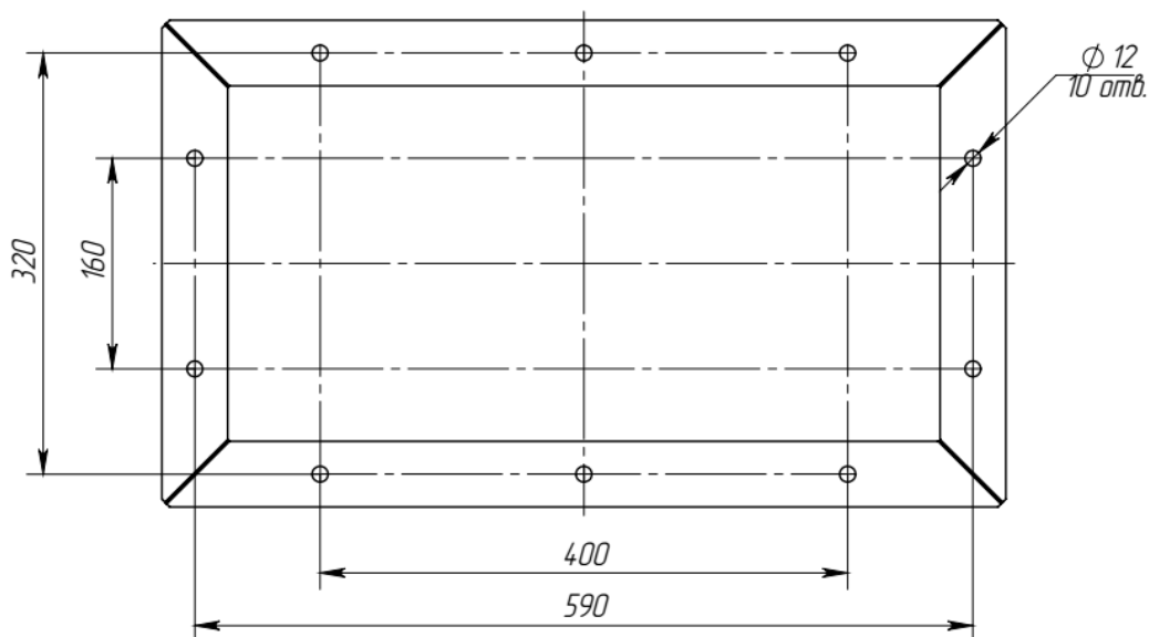
Рисунок 6 – Крепежные отверстия цоколя МПЧ (вид снизу)
