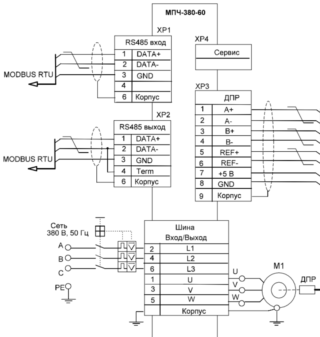
Рисунок 9 – Рекомендуемая схема подключения МПЧ
