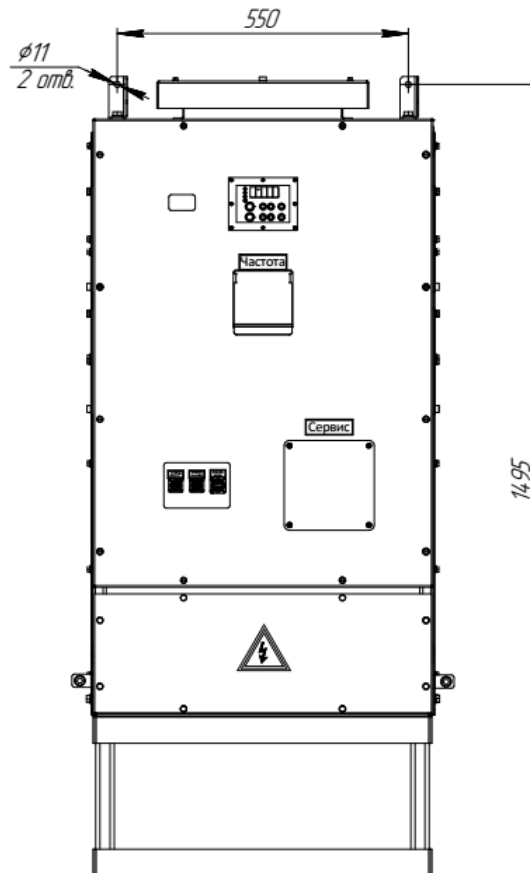
Рисунок 5 – Размеры крепежных отверстий для крепления к стене
