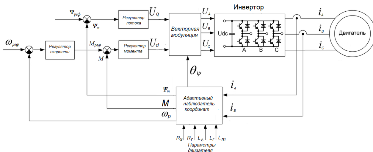
Рисунок 11– Структурная схема векторного управления асинхронным двигателем
