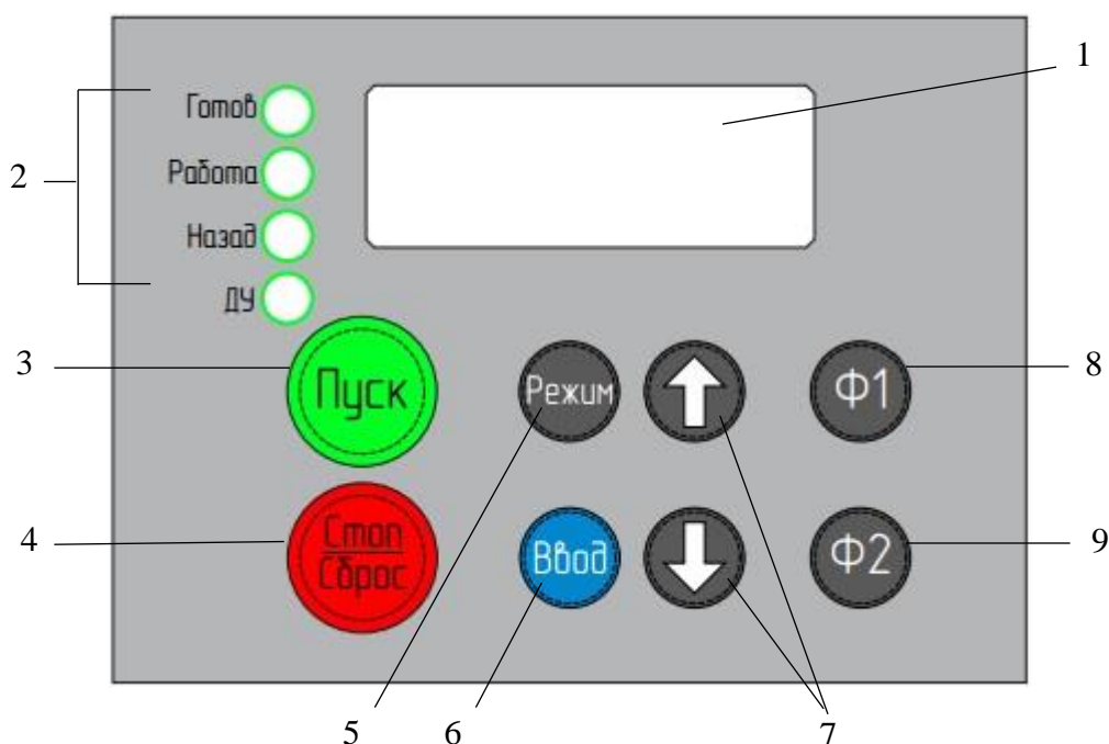
Рисунок 3 – Панель управления МПЧ-380-60В
