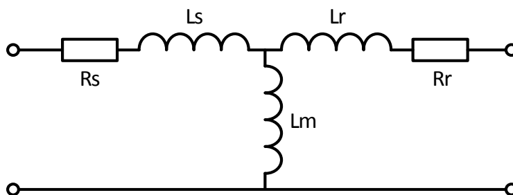
Рисунок 12 – Эквивалентная схема замещения асинхронного двигателя
