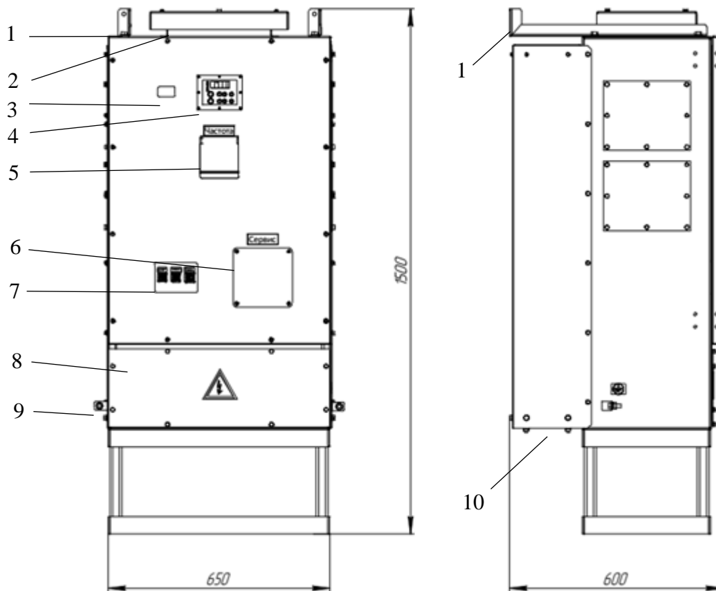
Рисунок 1 – Внешний вид МПЧ
